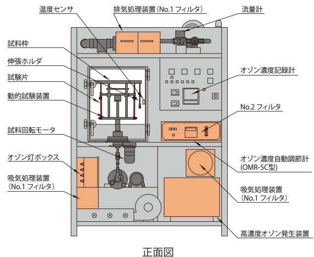
正面図
